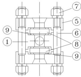
本體剖面圖
