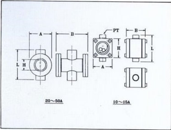
尺寸材質及一般規格表適用: SG300型 (暫無生產)
