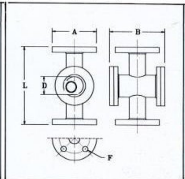
尺寸表: mm 適用SG200型
