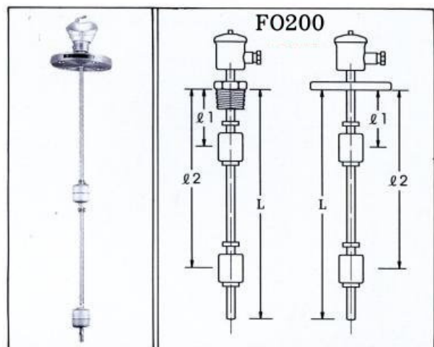
一般規格表：FO200型
