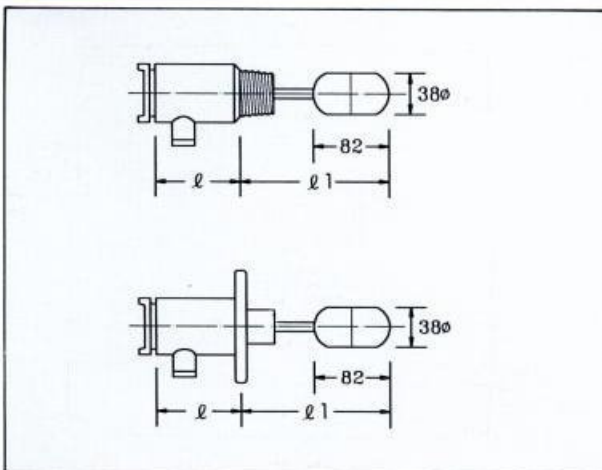
FO100 外形圖
